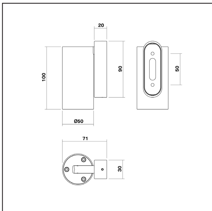
Dimensions
